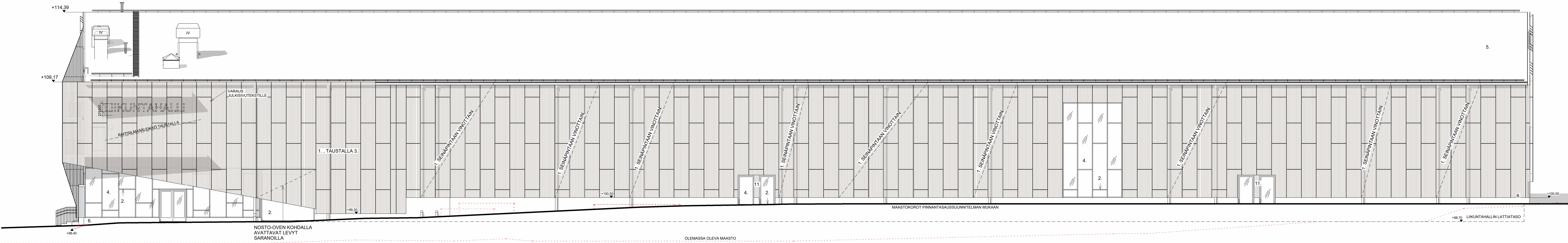
JULKISIVU POHJOISEN 1 : 100
